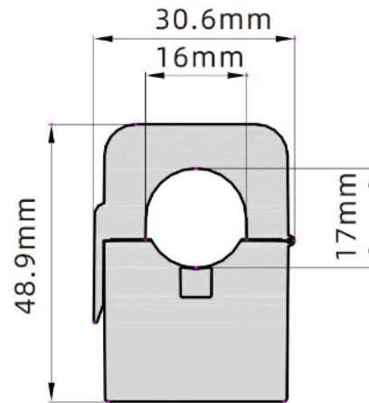
100A CT
