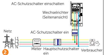
AC-Schutzschalter einschalten
