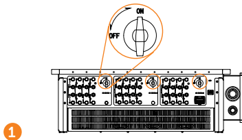
DC-Schalter einschalten
