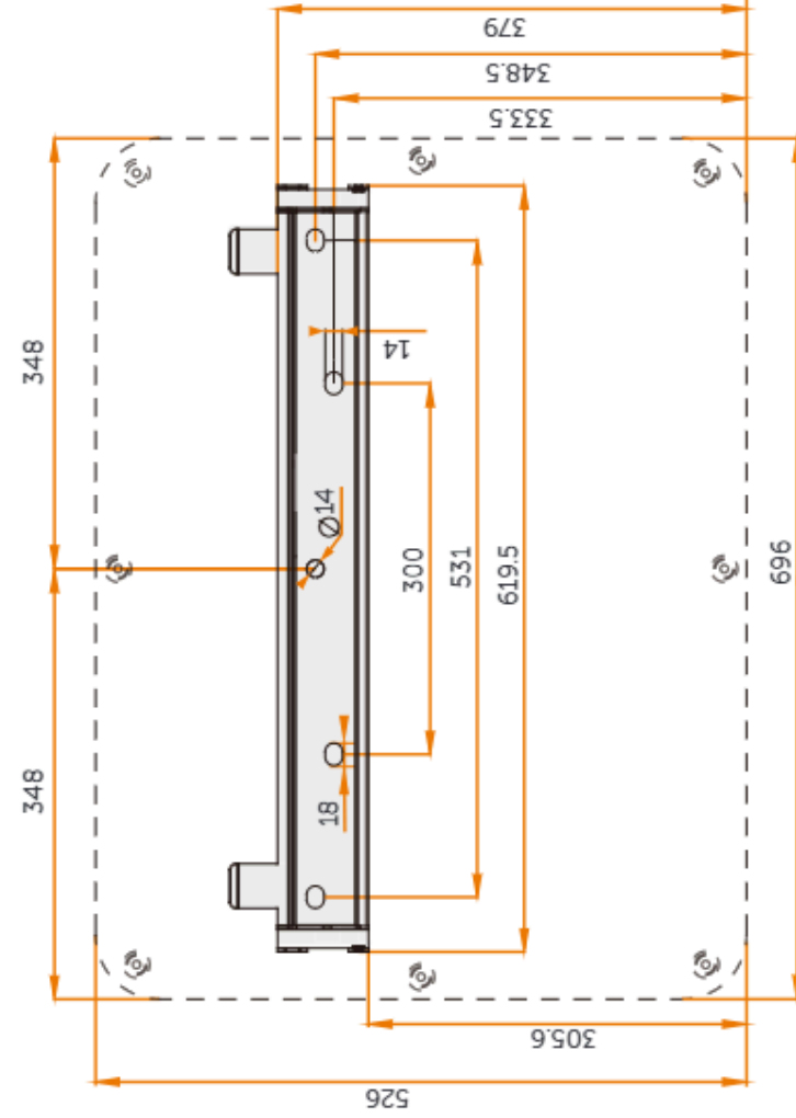
Abbildung 7-4 Abmessungen 2 (Einheit: mm)
