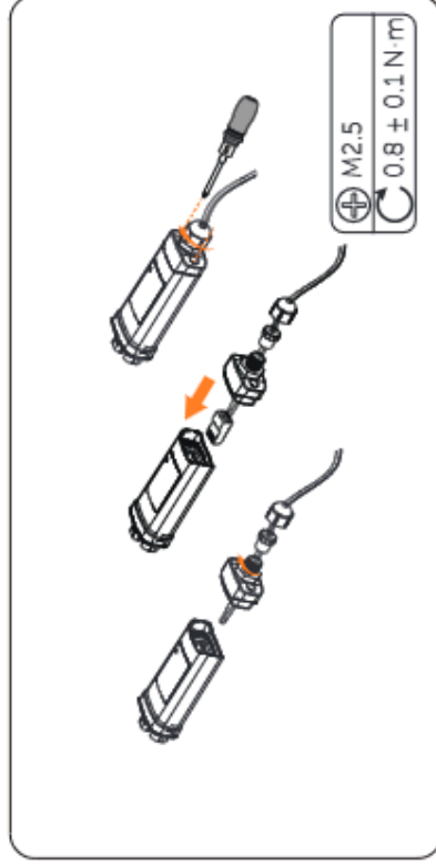
Abbildung 8-71 Den Dongle montieren
