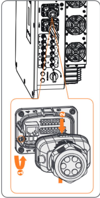
Abbildung 8-52 COM 2-Klemme demonstrieren
