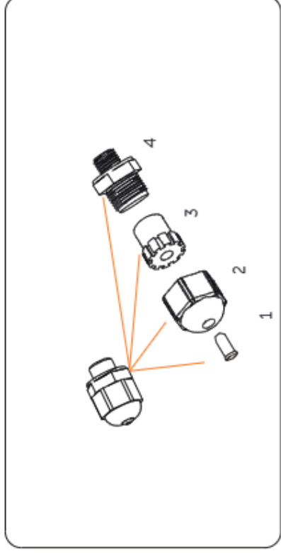
Abbildung 8-70 Den wasserdichten Steckverbinder demontieren
