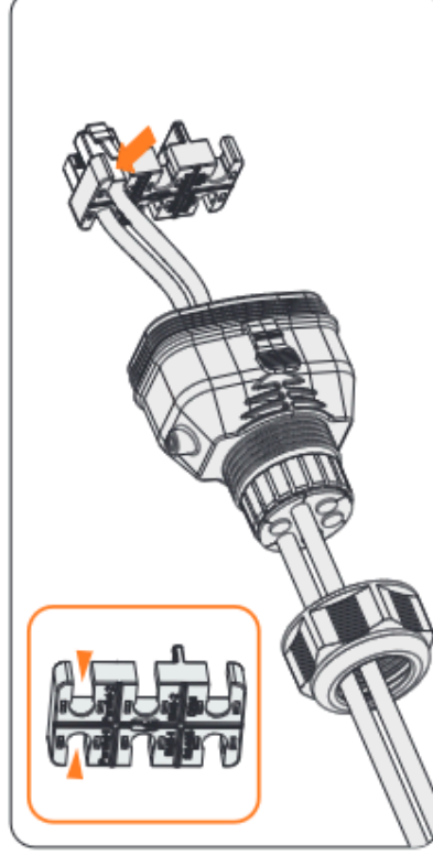
Abbildung 8-38 RJ45-Klemme an dem Kabelhalter anbringen
