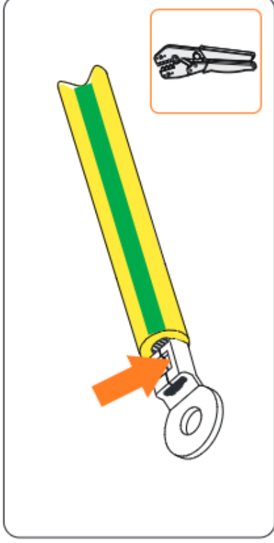
Abbildung 8-5 Das Kabel crimpen
