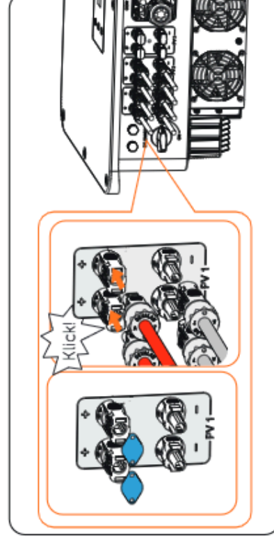
Abbildung 8-21 Das PV-Kabel anschließen
