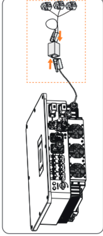
Abbildung 8-57 An Draht-Meter anschließen
