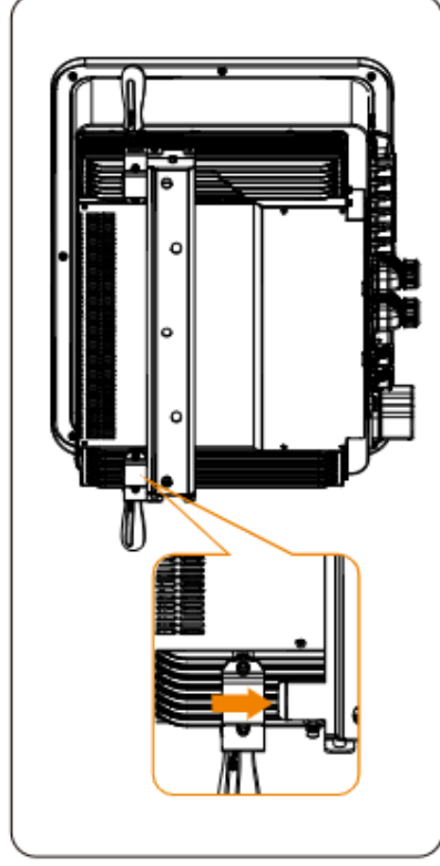
Abbildung 7-9 Wechselrichter aufhängen
