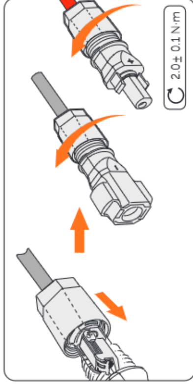
Abbildung 8-33 Die Kabelverschraubung festziehen
