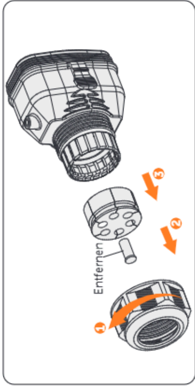
Abbildung 8-53 Den Steckverbinder demonstrieren
