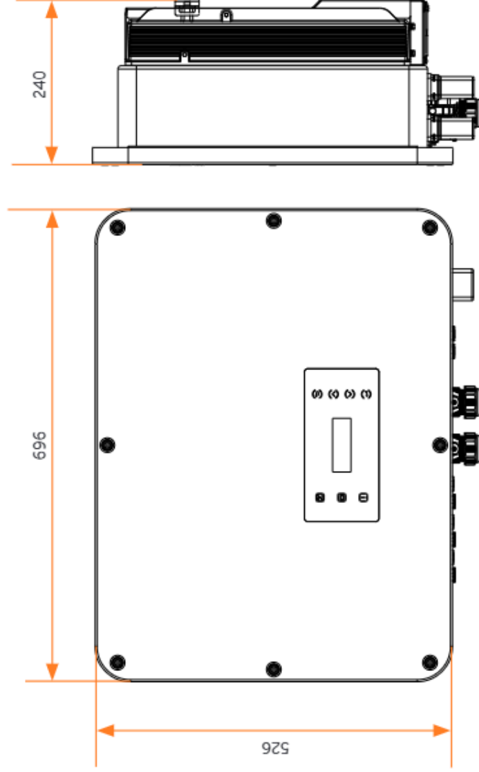
Abbildung 7-3 Abmessungen 1 (Einheit: mm)
