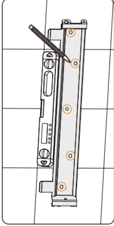
Abbildung 7-5 Die Löcher markieren
