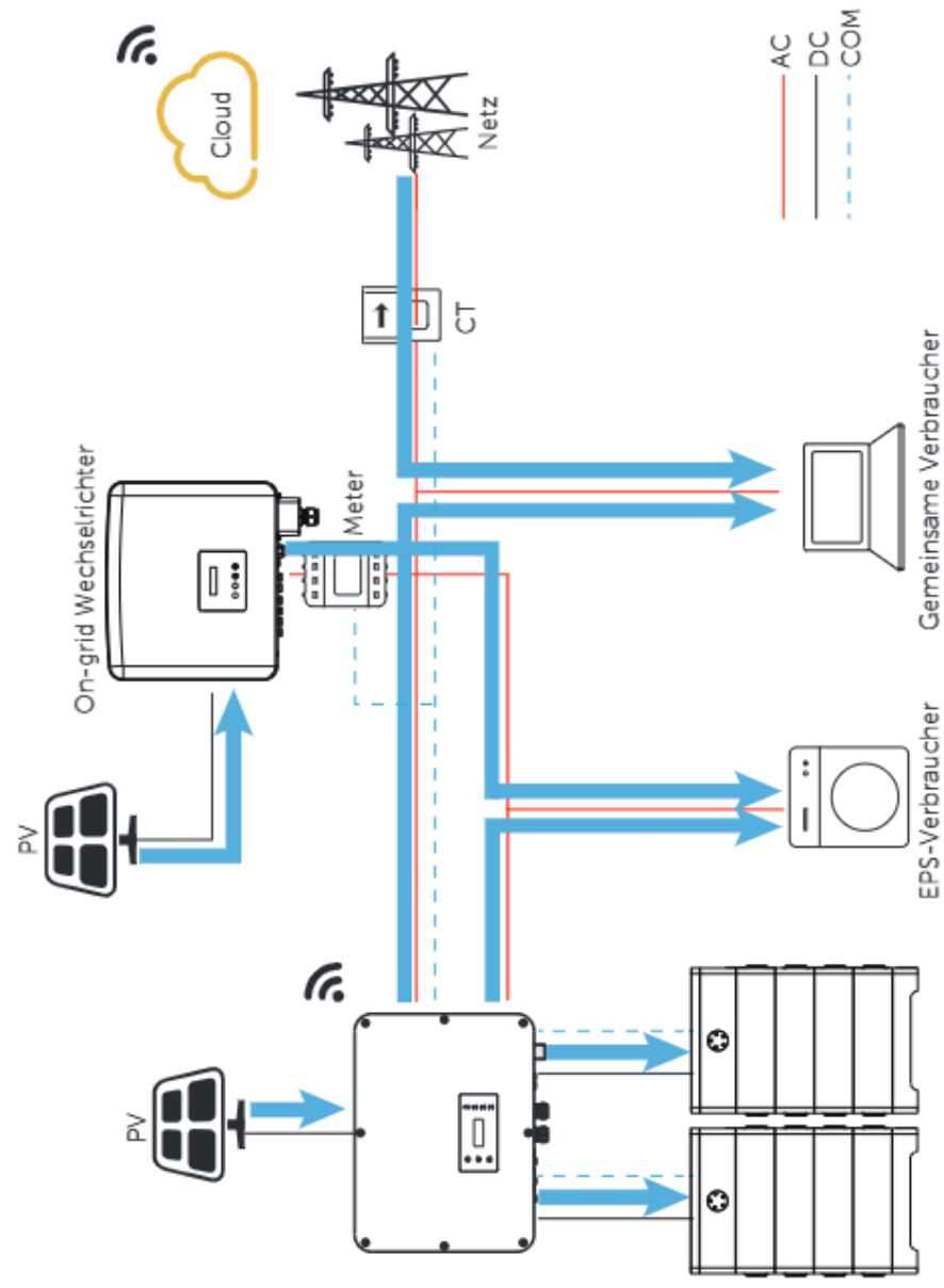
Abbildung 15-14 Stromfluss bei eingeschaltetem Netz und ausreichender PV-Leistung
