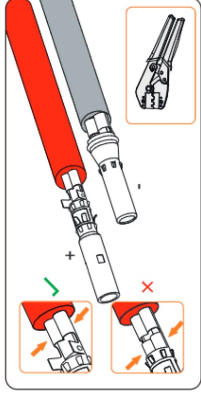
Abbildung 8-17 Die Klemme crimpen
