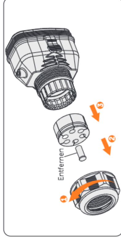
Abbildung 8-43 Den Steckverbinder demontieren
