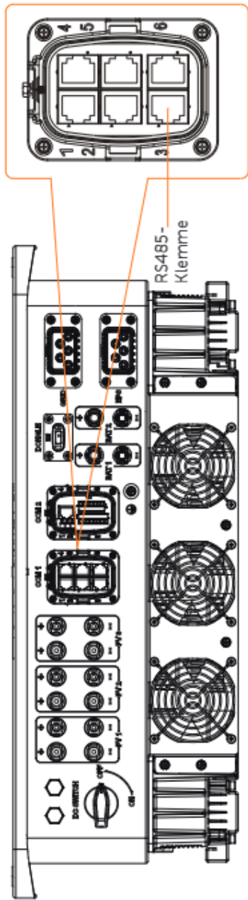
Abbildung 15-11 Anschlussklemme für DataHub
