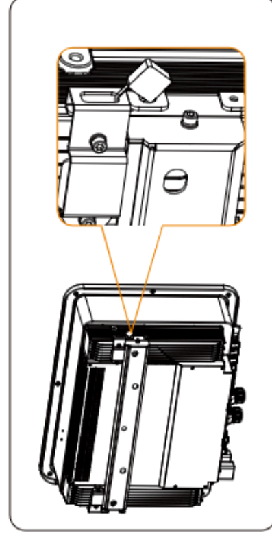
Abbildung 7-11 Den Wechselrichter verriegeln
