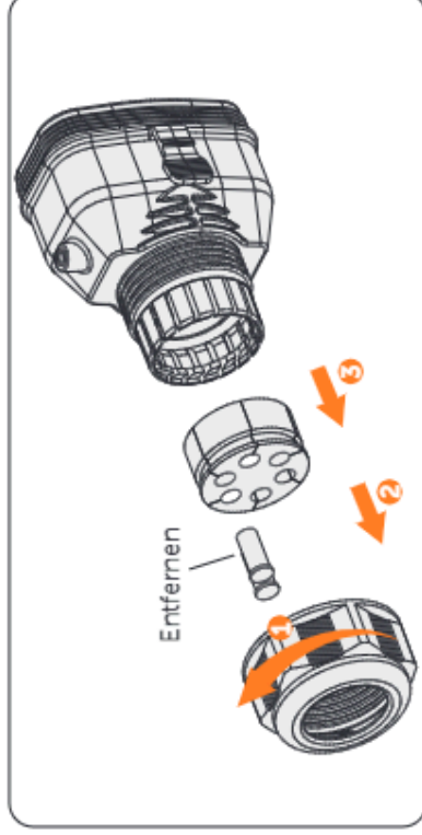
Abbildung 8-60 Den Steckverbinder demontieren
