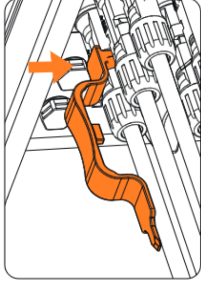
Abbildung 13-2 PV-Steckverbinder lösen
