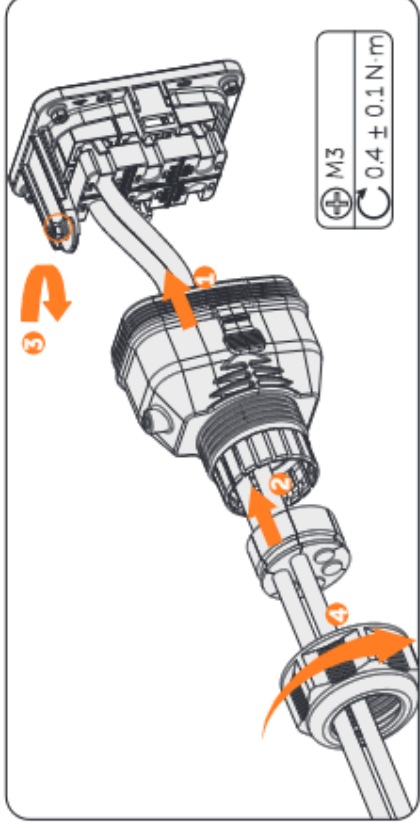
Abbildung 8-40 Den Steckverbinder sichern
