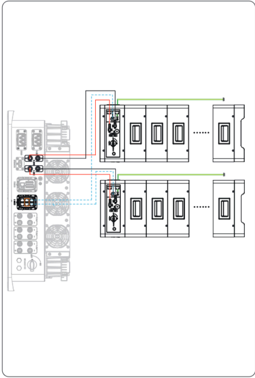
Abbildung 8-26 Detaillierter Anschlussplan 2
