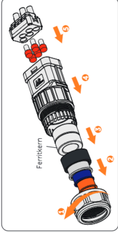
Abbildung 8-9 AC-Steckverbinder demontieren
