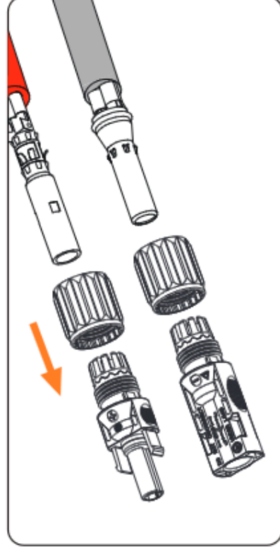
Abbildung 8-18 Das PV-Kabel einfädeln
