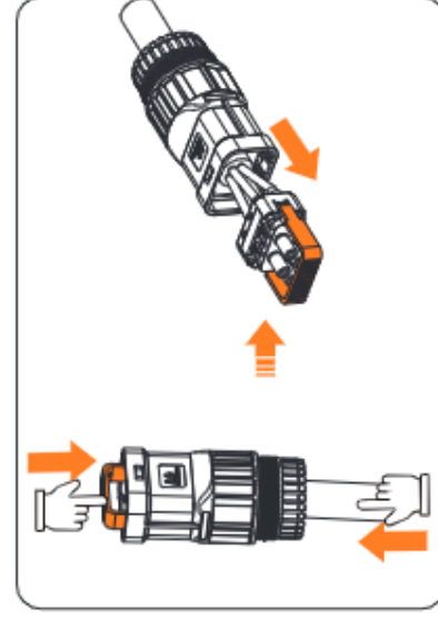
Abbildung 13-7 Den AC-Steckverbinder abtrennen
