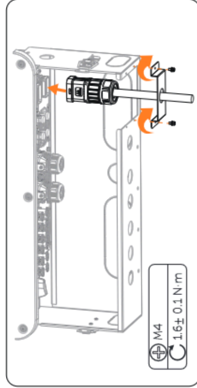
Abbildung 15-30 AC-Steckverbinder installieren
