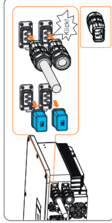
Abbildung 8-13 Den AC-Steckverbinder am Wechselrichter installieren
