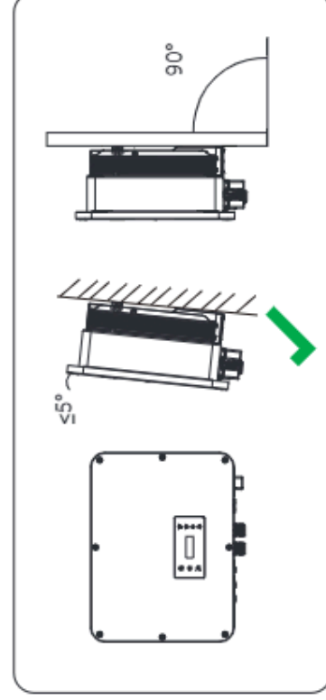
Abbildung 7-1 Korrekte Installation
