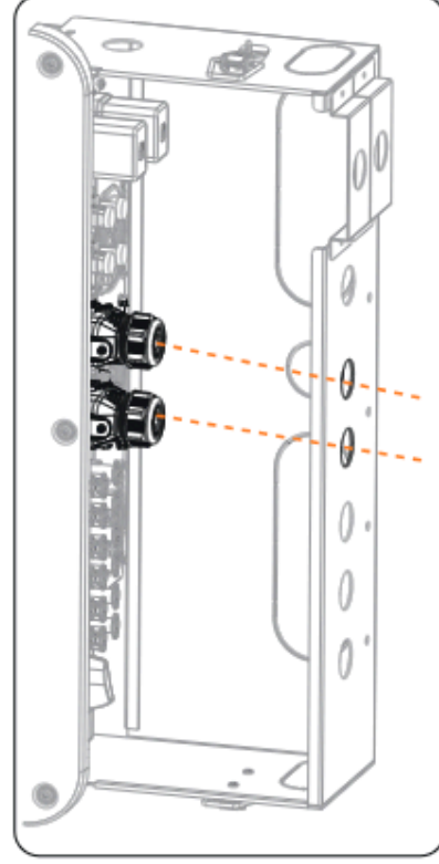
Abbildung 15-33 An COM-Klemme anschließen
