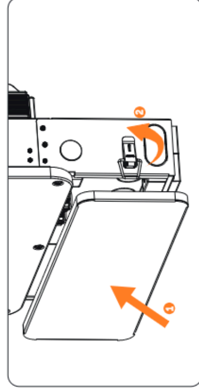
Abbildung 15-38 Frontplatte installieren
