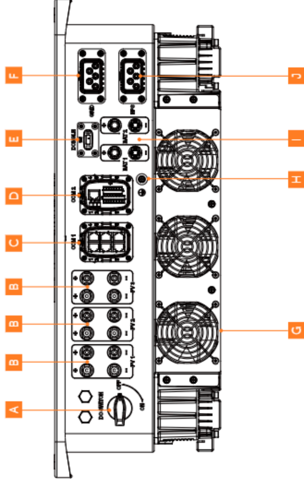
Abbildung 8-1 Klemmen des Wechselrichters
