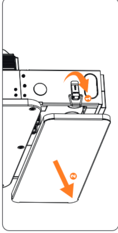
Abbildung 15-26 Die Frontplatte entfernen
