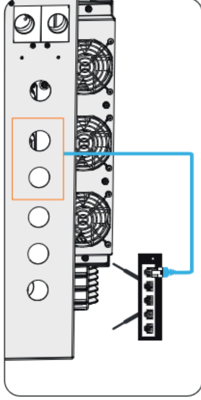
Abbildung 15-37 Dongle installieren
