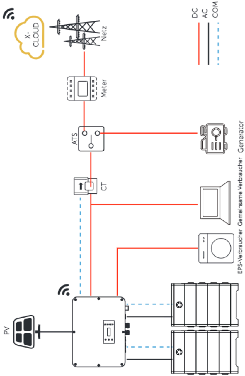
Abbildung 15-1 Schaltplan von ATS-Steuerung
