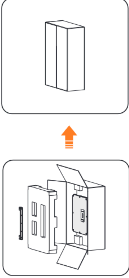
Abbildung 13-9 Den Wechselrichter verpacken
