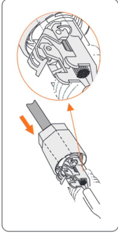
Abbildung 8-31 Das Batteriekabel einfädeln
