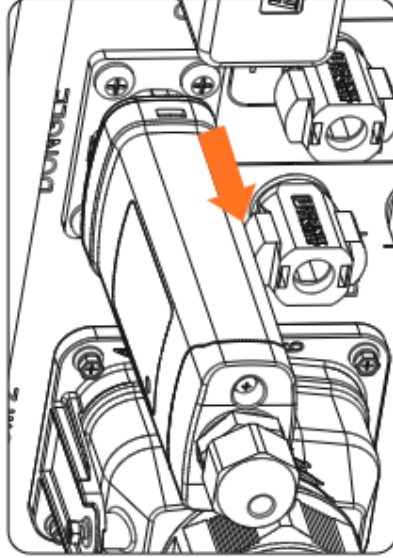
Abbildung 13-3 Den Dongle entfernen
