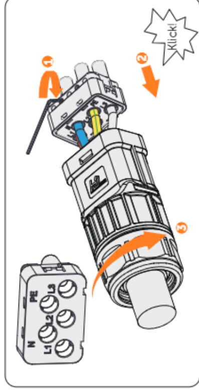
Abbildung 8-12 AC-Steckverbinder montieren
