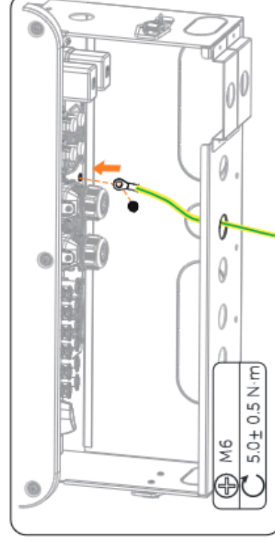
Abbildung 15-27 Das PE-Kabel anschließen
