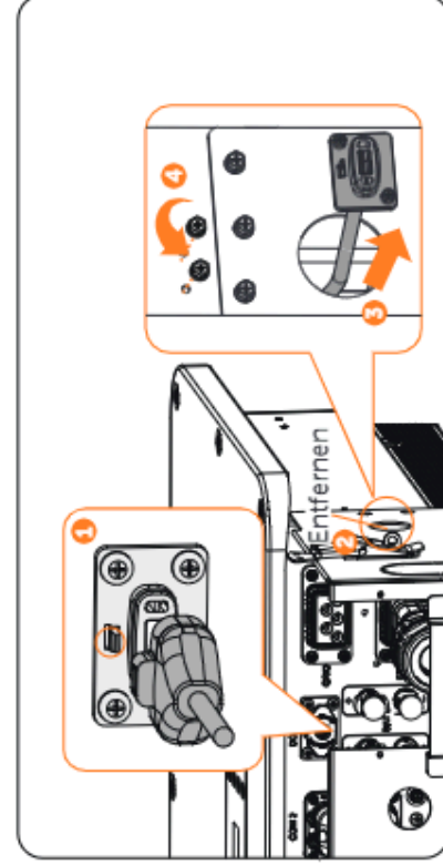
Abbildung 15-34 WiFi-Verbindungskabel installieren
