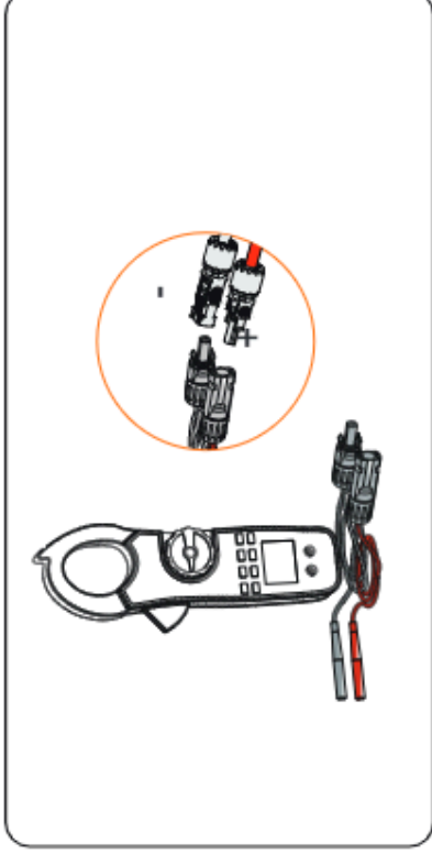
Abbildung 8-20 Die Spannung von PV-Steckverbindern messen
