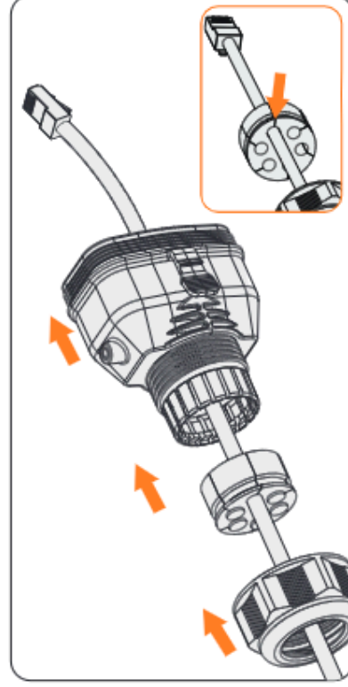
Abbildung 8-44 Kabel einfädeln
