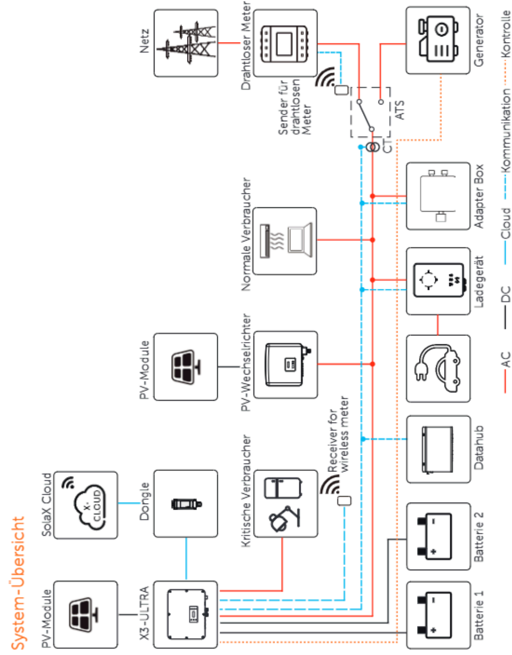
Abbildung 3-17 System-Übersichtsdiagramm
