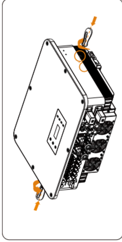
Abbildung 7-8 Handgriffe anbringen
