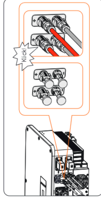
Abbildung 8-34 Batterie-Steckverbinder anschließen
