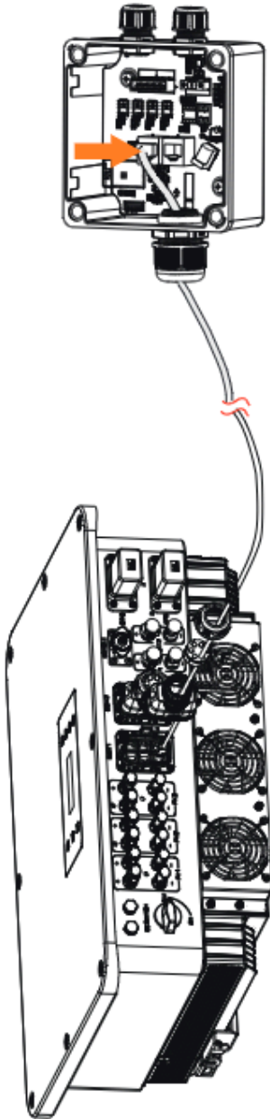
Abbildung 15-6 An die Adapterbox anschließen
