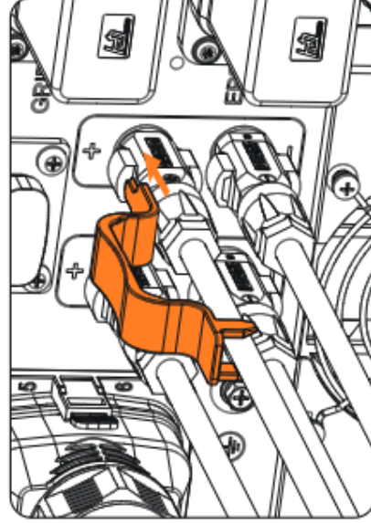
Abbildung 13-4 Batterie-Steckverbinder entfernen
