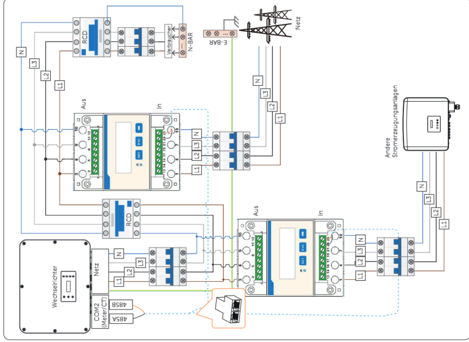
Abbildung 8-49 Meter-Anschlussplan 2
