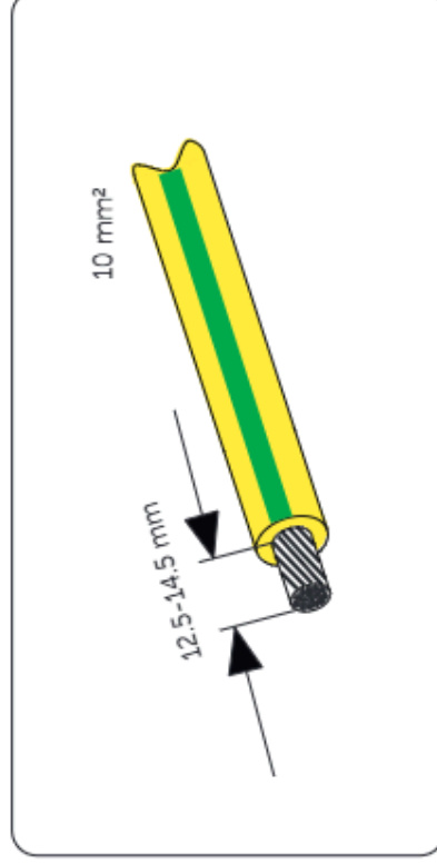
Abbildung 8-3 Das PE-Kabel abisolieren
