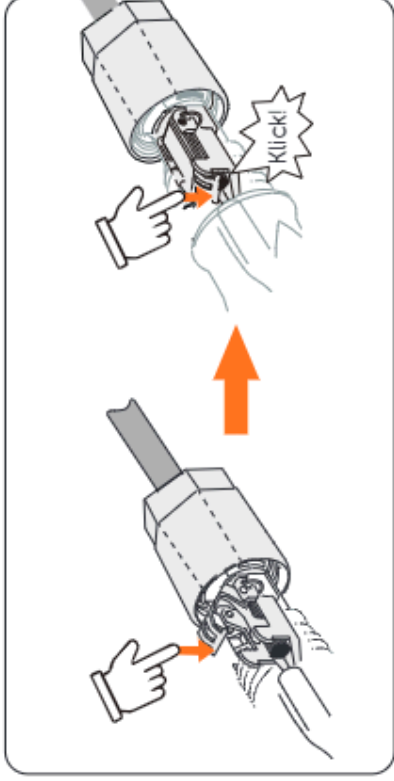
Abbildung 8-32 Die Feder nach unten drücken
