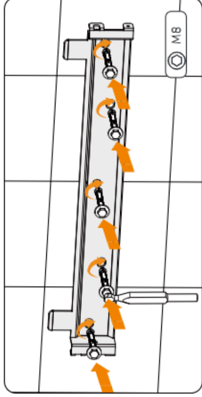
Abbildung 7-7 Die Schrauben einsetzen
