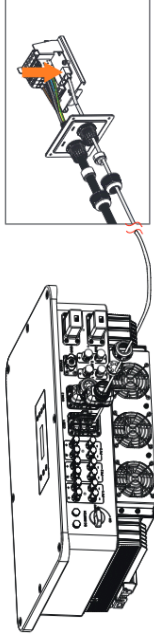
Abbildung 15-9 An EV-Ladegerät anschließen
