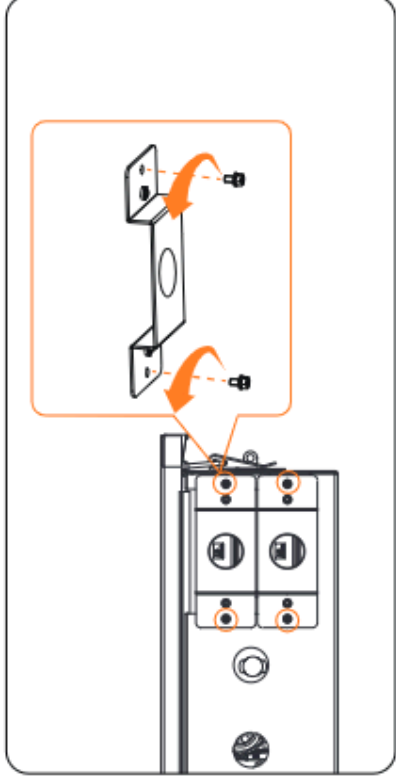
Abbildung 15-28 Die Schrauben der Kabelabdeckung lösen
