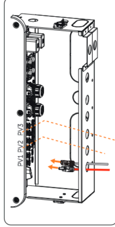
Abbildung 15-31 Das PV-Kabel anschließen
