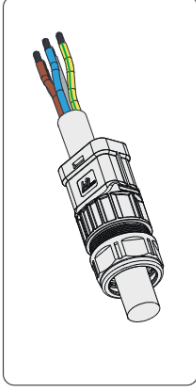
Abbildung 8-10 Netzkabel einfädeln
