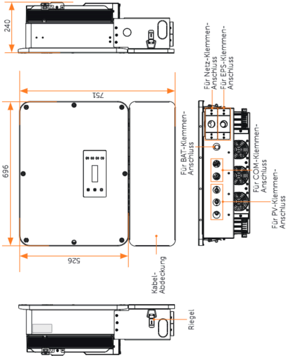
Abbildung 15-23 Erscheinungsbild mit Kabelabdeckung (Einheit: mm)
