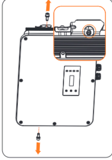
Abbildung 13-8 Die M5-Schrauben herausdrehen
