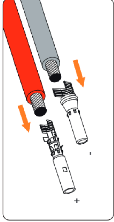
Abbildung 8-16 PV-Pin-Kontakt einsetzen
