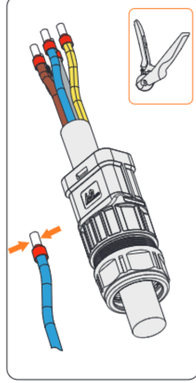
Abbildung 8-11 Das Kabelende abisolieren und crimpen
