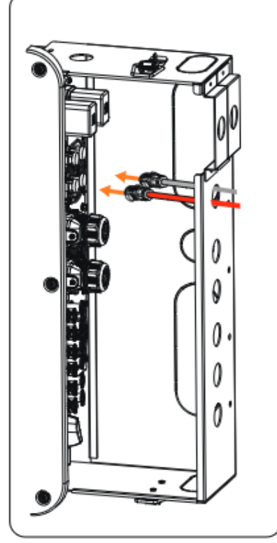
Abbildung 15-32 Batteriestromkabel anschließen
