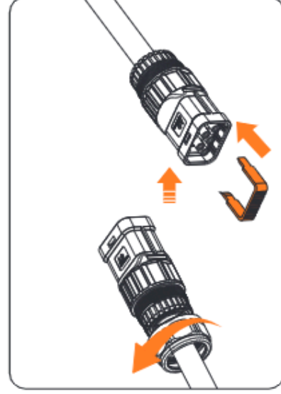
Abbildung 13-6 Die Überwurfmutter entfernen
