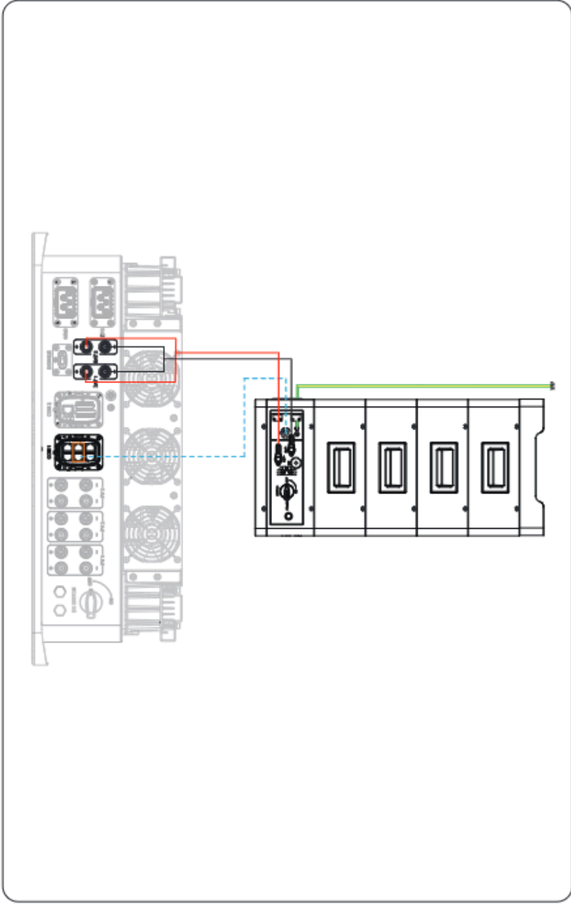
Abbildung 8-28 Detaillierter Anschlussplan 3
