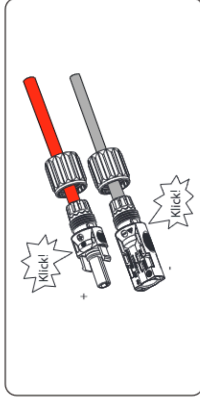
Abbildung 8-19 Das PV-Kabel sichern
