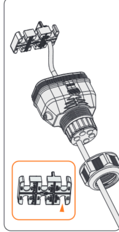
Abbildung 8-45 RJ45-Klemme an dem Kabelhalter anbringen
