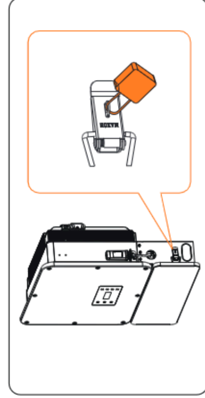
Abbildung 15-39 Schlösser installieren
