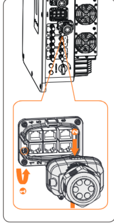
Abbildung 8-35 Das Gehäuse des Steckverbinders entfernen
