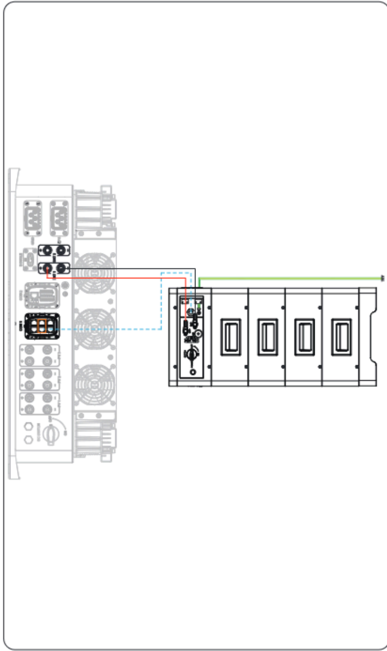
Abbildung 8-23 Batterie-Anschlussplan 1
