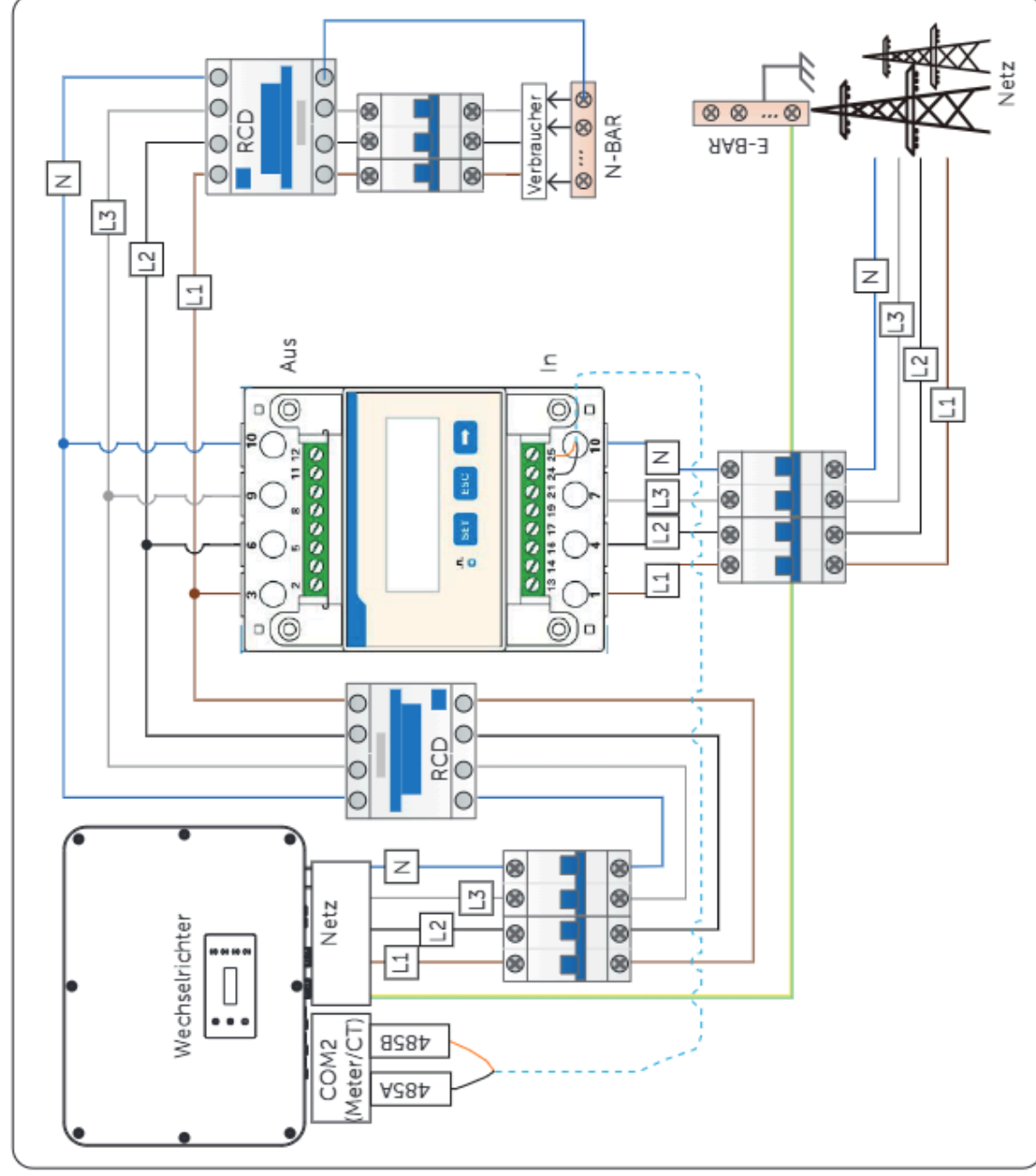
Abbildung 8-48 Meter-Anschlussplan 1
