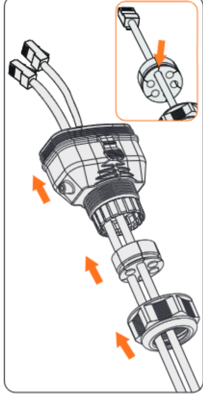
Abbildung 8-37 Kabel einfädeln
