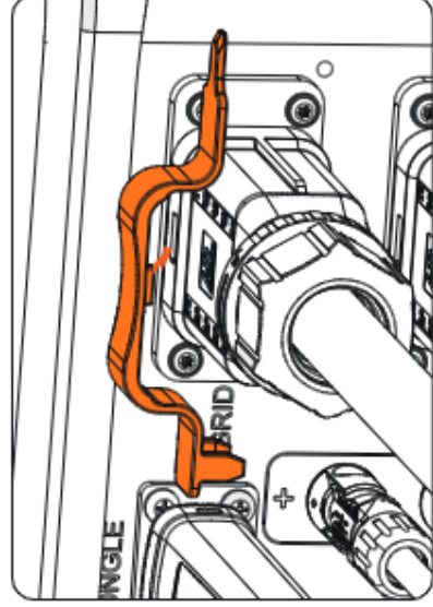
Abbildung 13-5 AC-Steckverbinder entfernen
