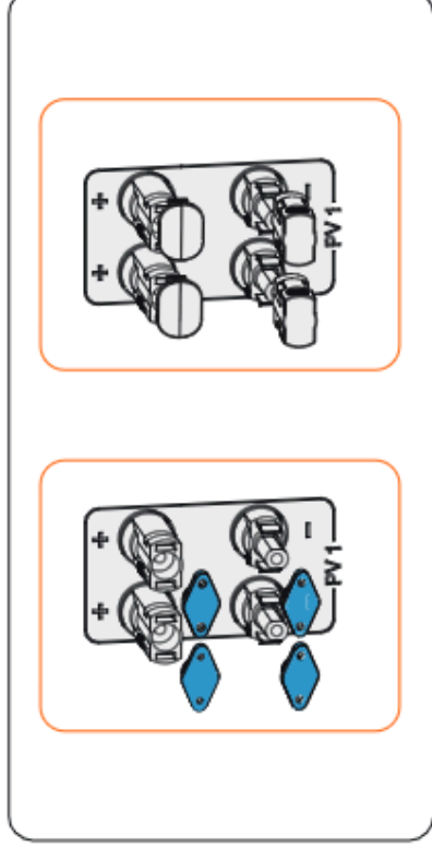
Abbildung 8-22 Die staubdichten Schnallen anschließen
