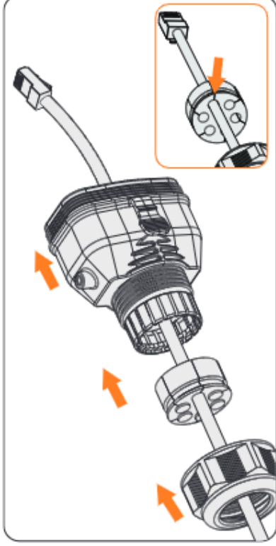
Abbildung 8-54 Kabel einfädeln
