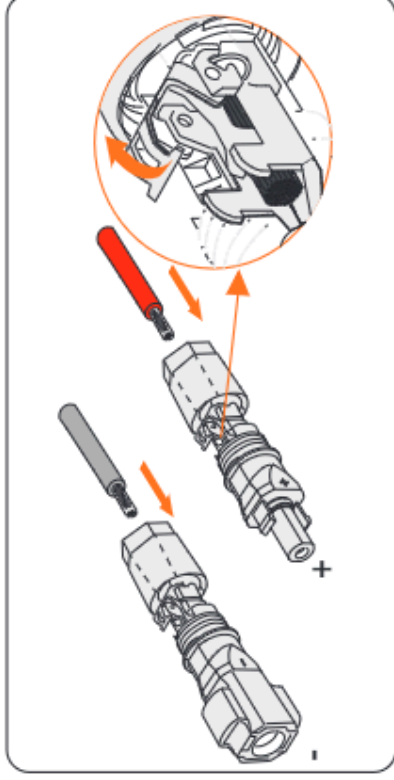
Abbildung 8-30 Die Feder öffnen
