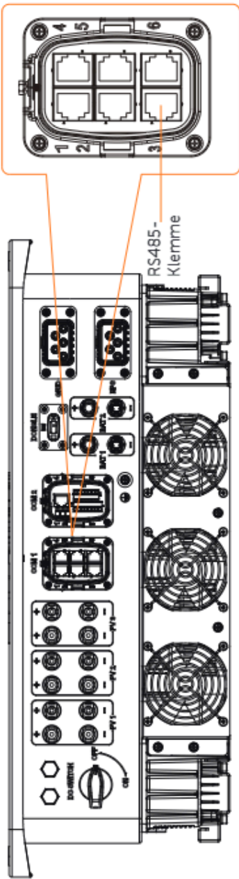
Abbildung 15-5 Anschlussklemme für Adapter Box
