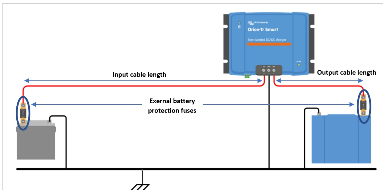
Abbildung 6: Kabel- und Sicherungsempfehlungen
