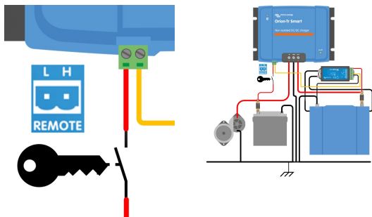
Abbildung 4: Anschlussplan für die Übersteuerung der Motorabschaltungserkennung
