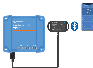
Die Verbindung mit der VictronConnect-App erfolgt über ein Bluetooth Smart Dongle VE.Direct.
