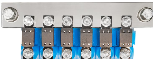
Stapelsicherungshalter mit 6-poliger Hochstromsammelschiene (Kupfer 40 x 5 mm)
