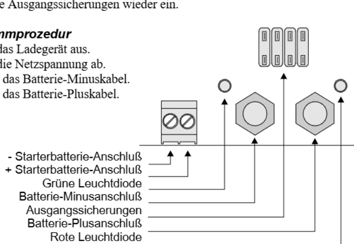
Abbildung 3. Lage der Batterie- Anschlüsse
