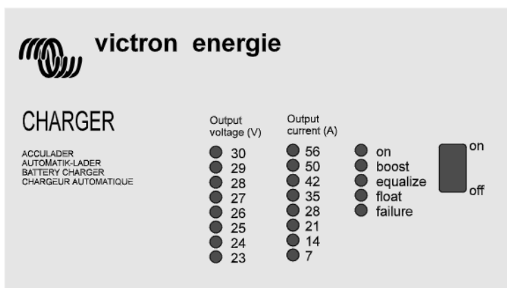
Abbildung 5. Beispiel der Frontplatte eines Titan-Ladegeräts
