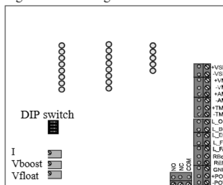
Abbildung 7. Lage des DIP-schalters und der Potentiometer
