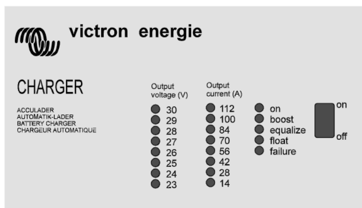
Abbildung 5. Beispiel der Frontplatte eines Skylla-TG-Ladegeräts
