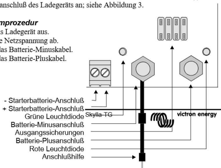
Abbildung 3. Lage der Batterie- Anschlüsse
