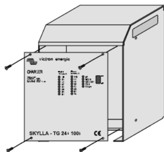
Abbildung 6. Entfernen der Frontplatte
