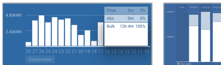
System verbringt die gesamte Zeit im Konstantstrom mit Aufgliederung der Ladephasen - System im Konstantstrom und in der Konstantspannung
