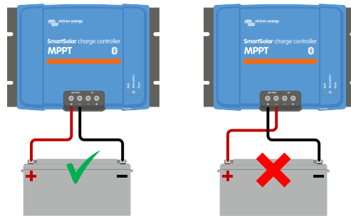
Beispiele für richtige und falsche (vertauschte) Batteriepolartität
