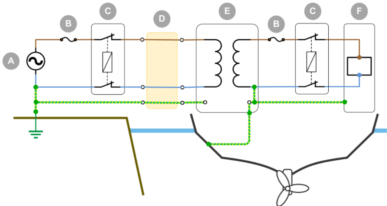
Verkabelungsbeispiel für einen auf einem Schiff installierten Trenntransformator, der an Landstrom angeschlossen ist.
